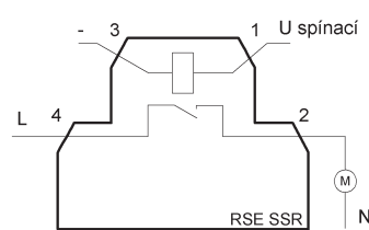
Příklad zapojení
